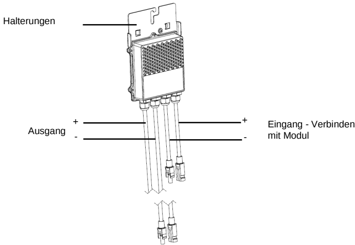
Abbildung 1: Leistungsoptimiereranschlüsse
