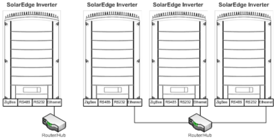
Anschluß einzelner Wechselrichter
