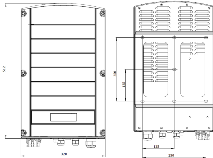
Abbildung 28: Dreiphasen-Wechselrichter mit Typ 1 Halterung - Vorder- und Rückansicht
