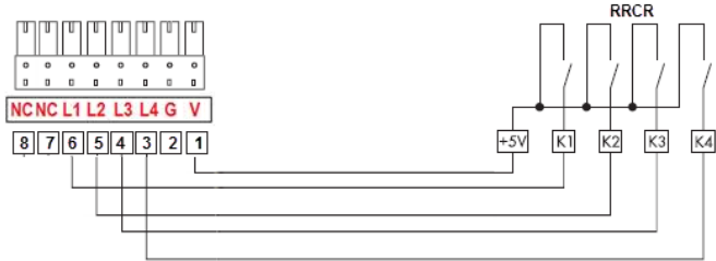
Abbildung 39 – Wechselrichter – FRSE-Anschluss
